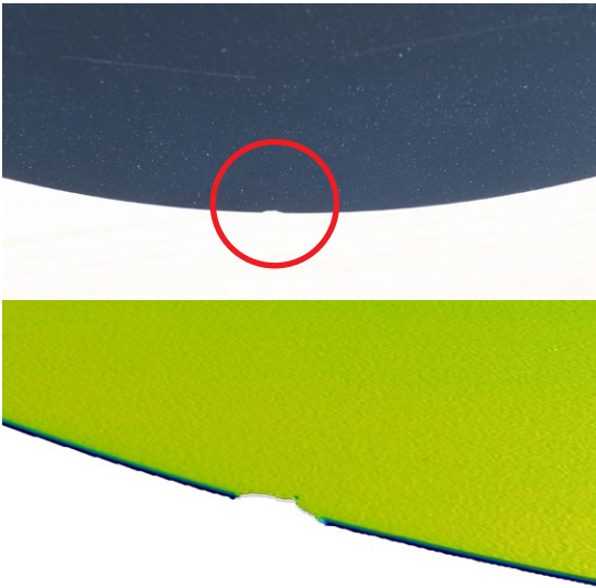
Die chipping inspection
